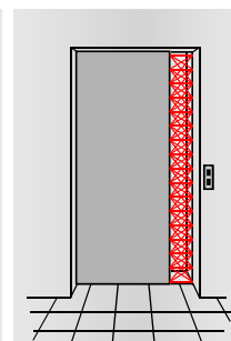
BARRIERA RAGGI INFRAROSSI INFRAROSSA INGRESSO/USCITA CABINA PER IL MASSIMO LIVELLO DI SICUREZZA IN/OUT BOX FOR THE HIGHEST LEVEL SAFETY
