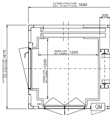
STRUTTURA METALLICA METALLIC SHAFT-TOWER TELESCOPIC DOORS
