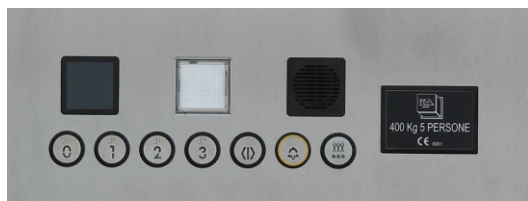
PULSANTIERA DI BORDO PUSH-BUTTON PANEL BOARD
